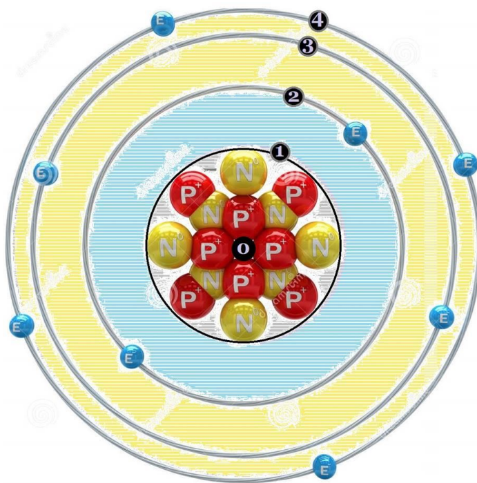
Structure atomique :
